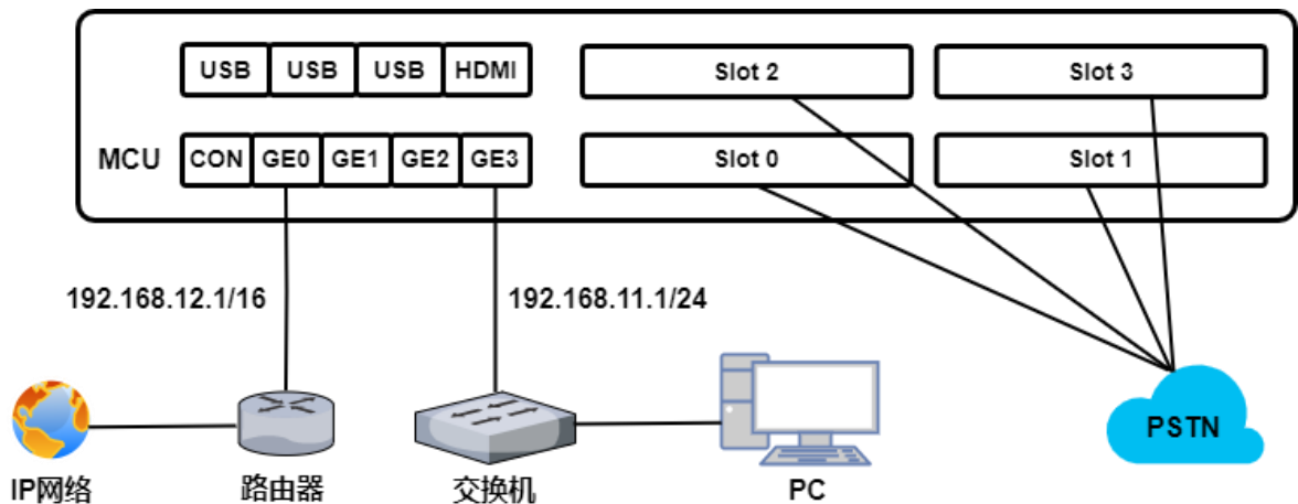
图 2.3 网络连接图
