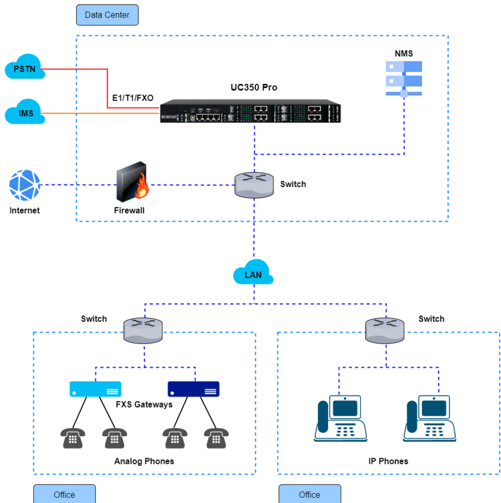
图 1-2-1 UC350 Pro 应用场景
